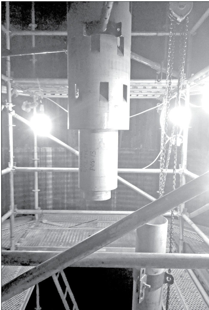
Работы с применением лесов Layher в варочной установке производства целлюлозы
